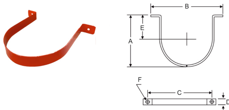
Рисунок 21 - Монтажная скоба
