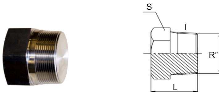
Рисунок 30 - Заглушка для установки в муфту соединения РВД
