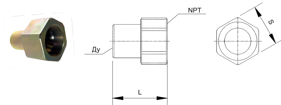
Рисунок 26 - Муфта-переходник для соединения штуцера ЗПУ с трубопроводом
