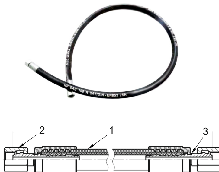
Рисунок 17 - Рукав высокого давления для пневмопуска модулей МПА-КД
