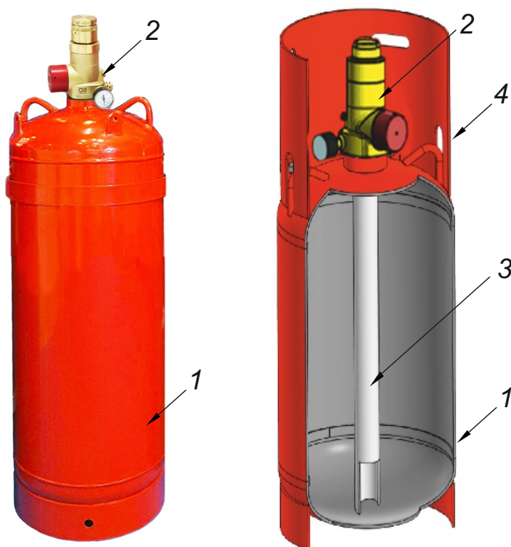
Рисунок 3 - Модуль газового пожаротушения МПА-КД (50-ХХ-50)
