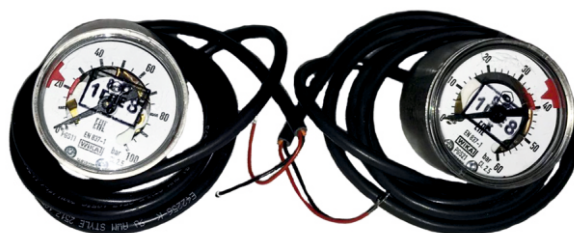
Рисунок 13 - Электроконтактный манометр
