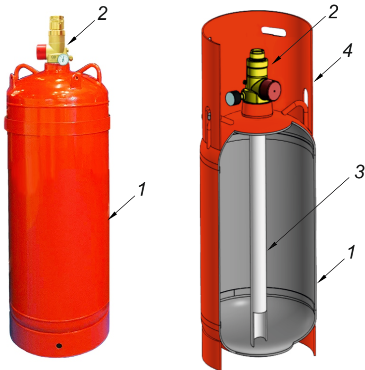
Рисунок 4 - Модуль газового пожаротушения МПА-КД (50-ХХ-33)
