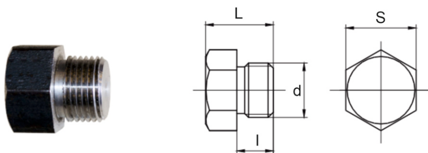
Рисунок 31 - Заглушка для установки в муфту СДУ
