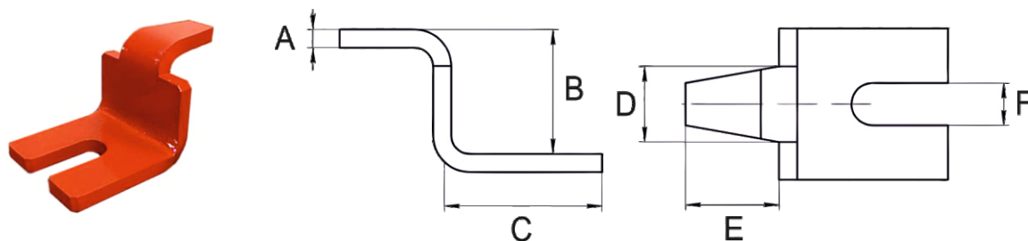
Рисунок 22 - Фиксатор крепления модулей к полу
