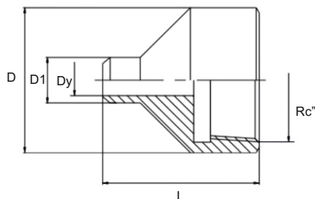
Рисунок 24 - Муфта переходная для соединения РВД с трубопроводом
