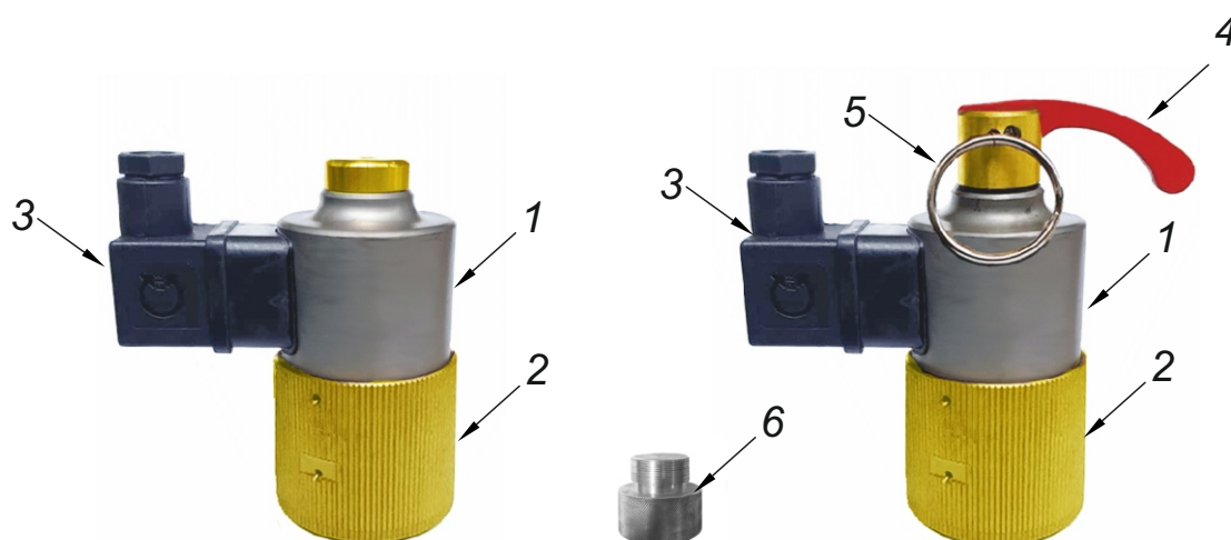
Рисунок 7 - Электромагнитный пуск ЭП-0418 (ЭПР-0418)
