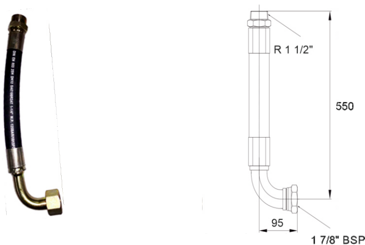
Рисунок 16 - Рукав высокого давления DN33
