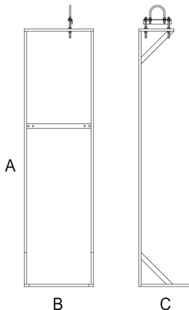
Рисунок 33 - Стойка для модулей МПА-КД
