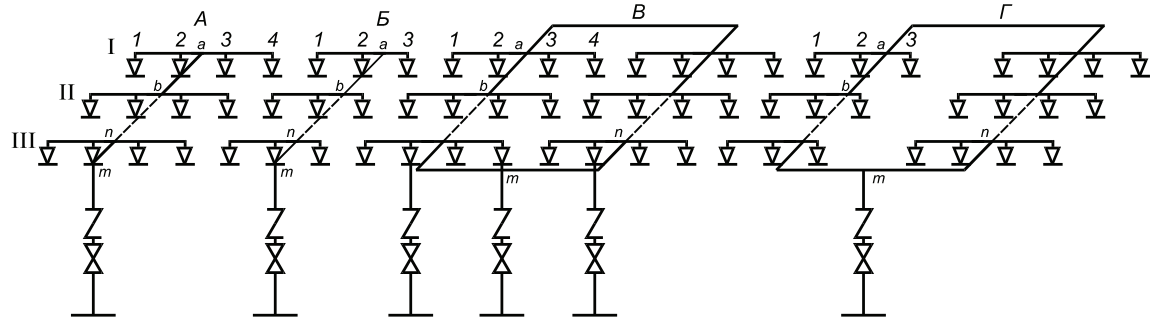
А — типичовая секция с симметричным расположением оросителей; Б — типичовая секция с несимметричным расположением оросителей; В — секция с симметричным кольцевым питающим трубопроводом; Г — секция с несимметричным кольцевым питающим трубопроводом; I, II, III — рядки распределительного трубопровода; а, b... n, m — узловые расчетные точки; 1, 2, 3, 4 — оросители
