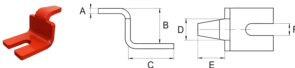
Рис. 19. Фиксатор крепления модулей к полу
