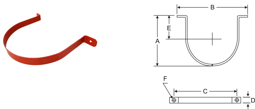
Рис. 18. Монтажная скоба
